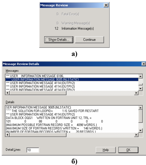
Рис.8.2. Панелі перегляду звіту про процес розв'язування крайової задачі
