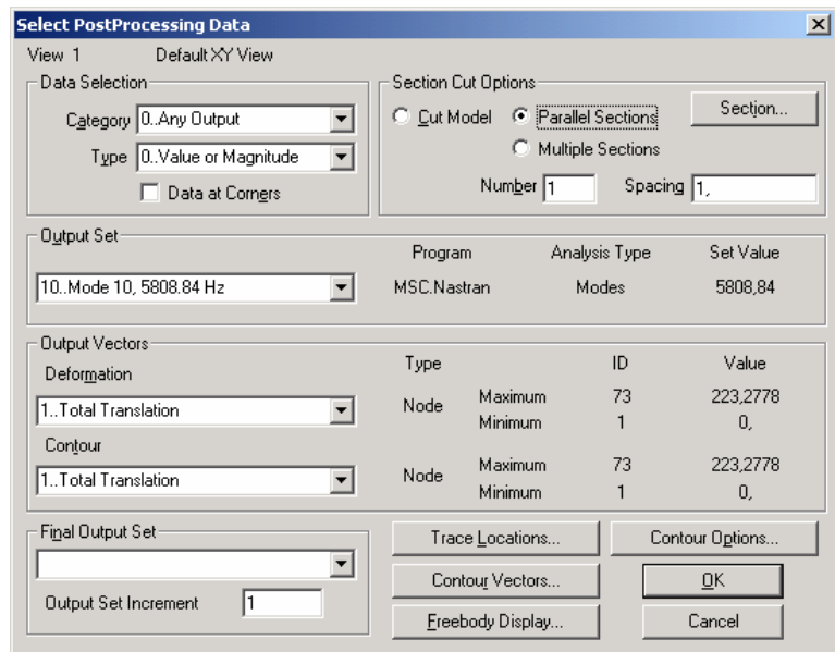
Рис.8.13. Діалогова панель призначення наборів та векторів результатів розрахунків для відображення у вигляді кольорових ізосмуг, ізоповерхонь та епюр
